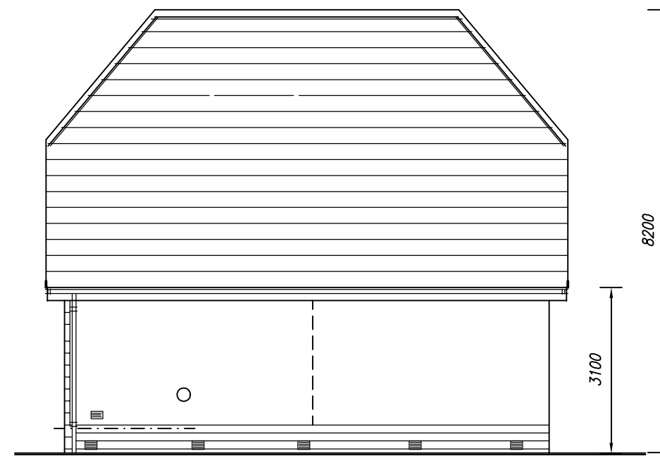
N.W. Elevation
