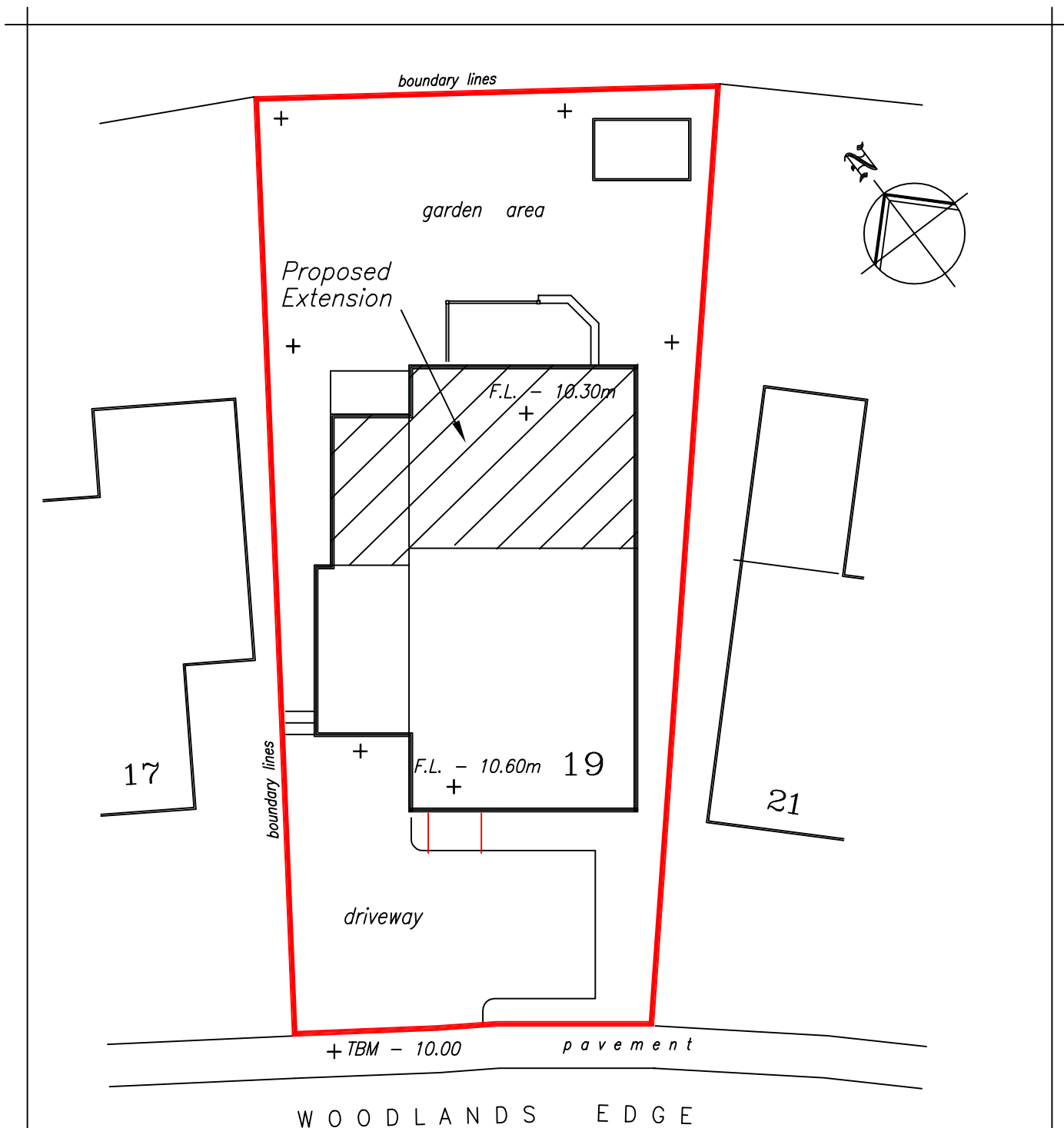
SITE LAYOUT PLAN :
