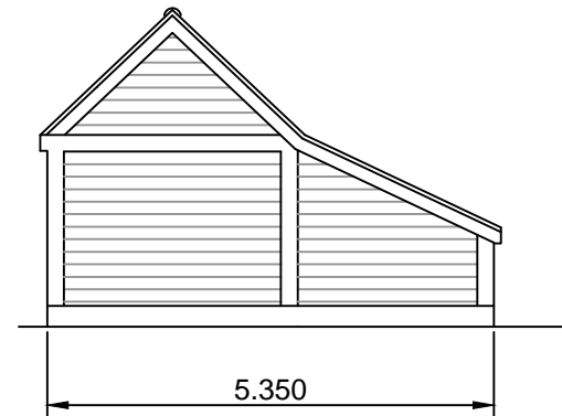
Right Elevation
