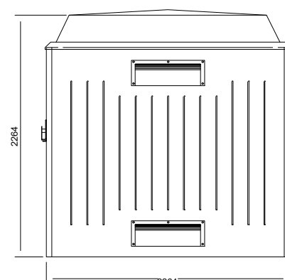
Elevation (D) (r/h side)
