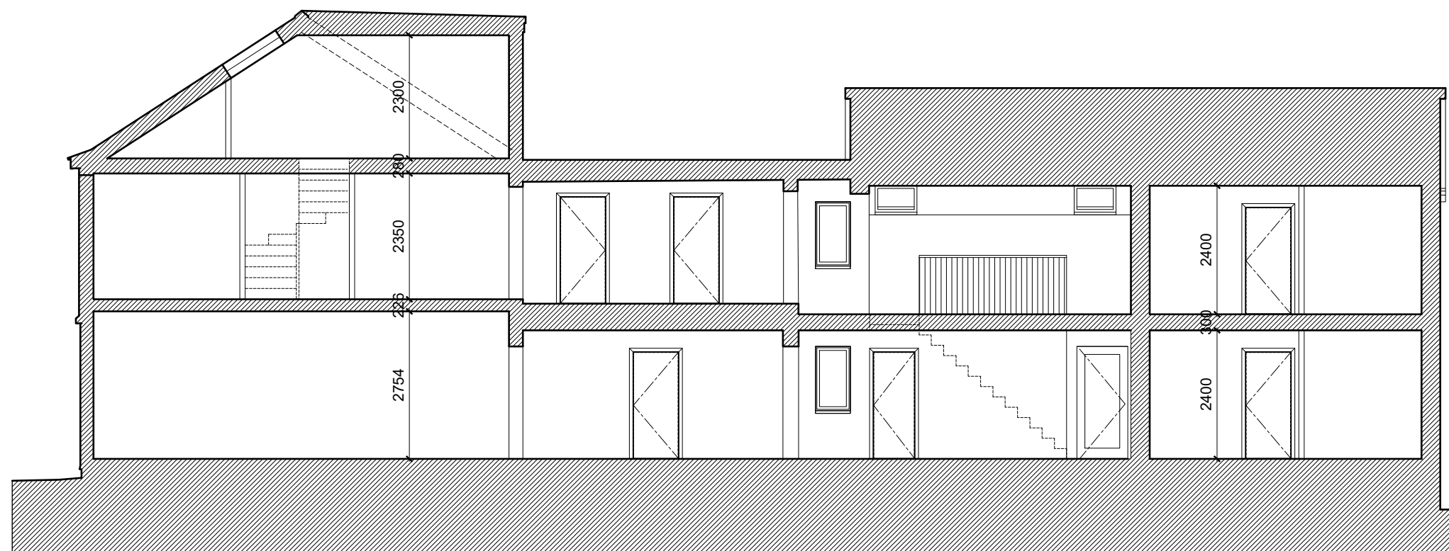
SECTION A-A
