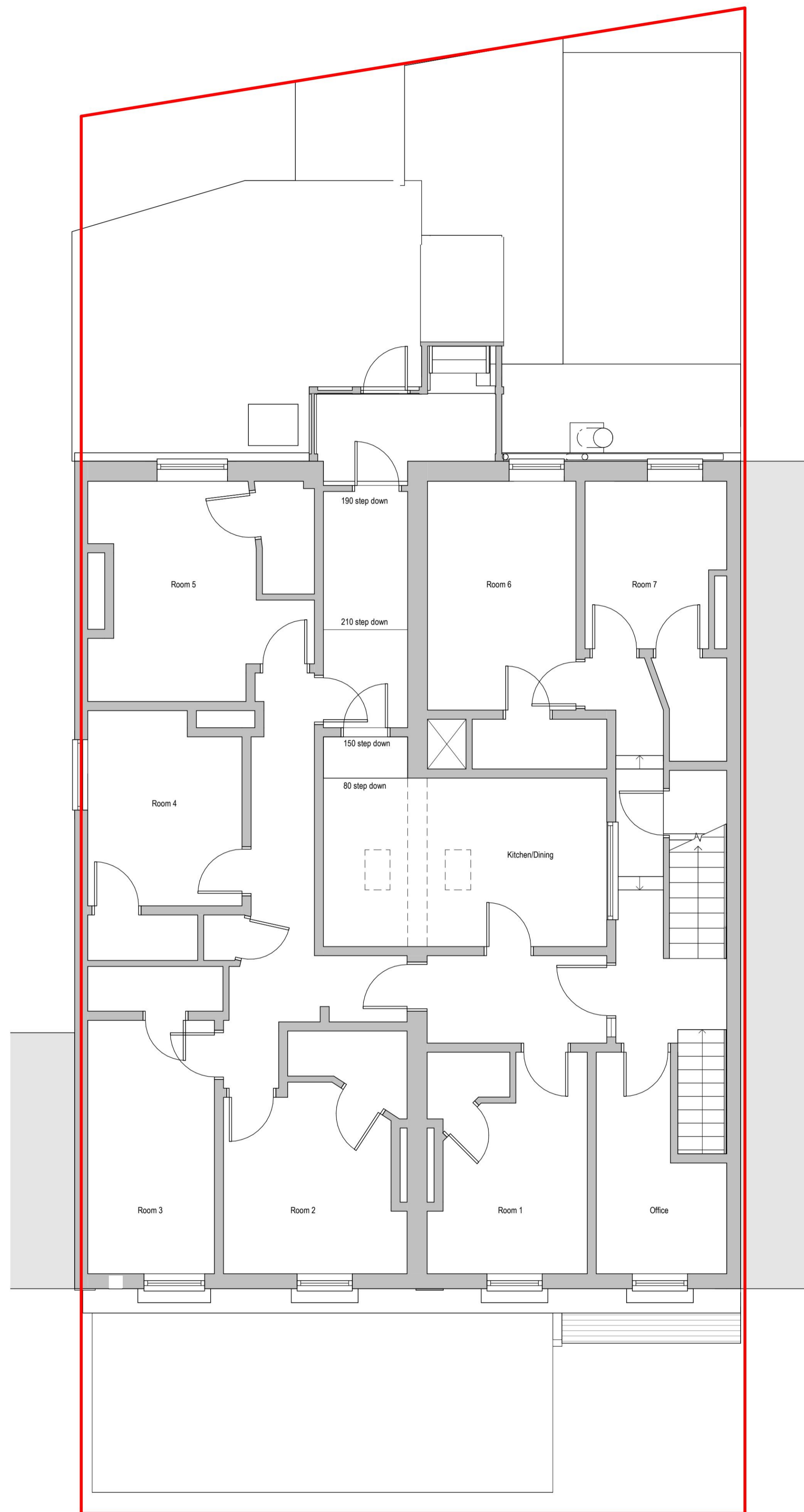
01 - GA Plan (Existing) 1 : 50
