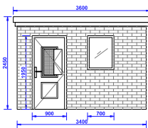
Right Elevation
