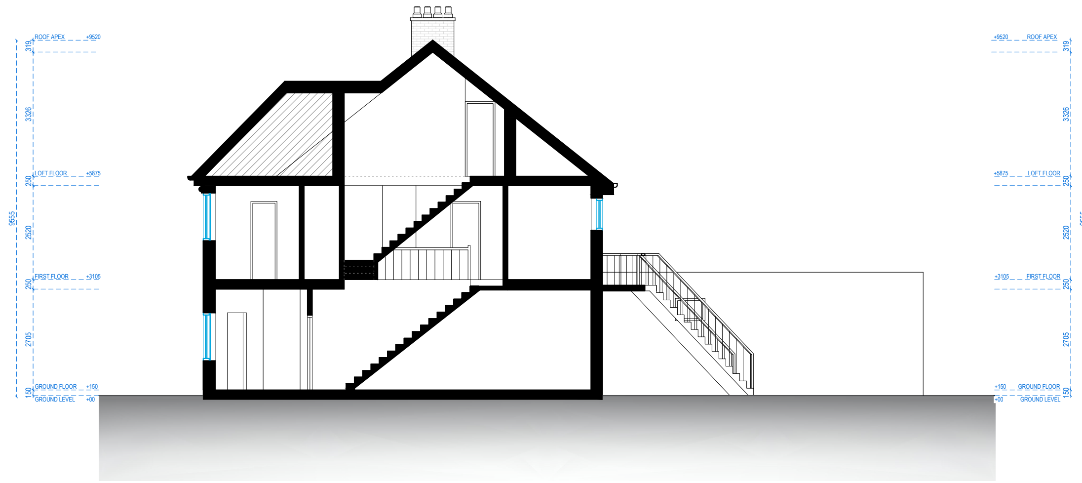
SECTION A.A
