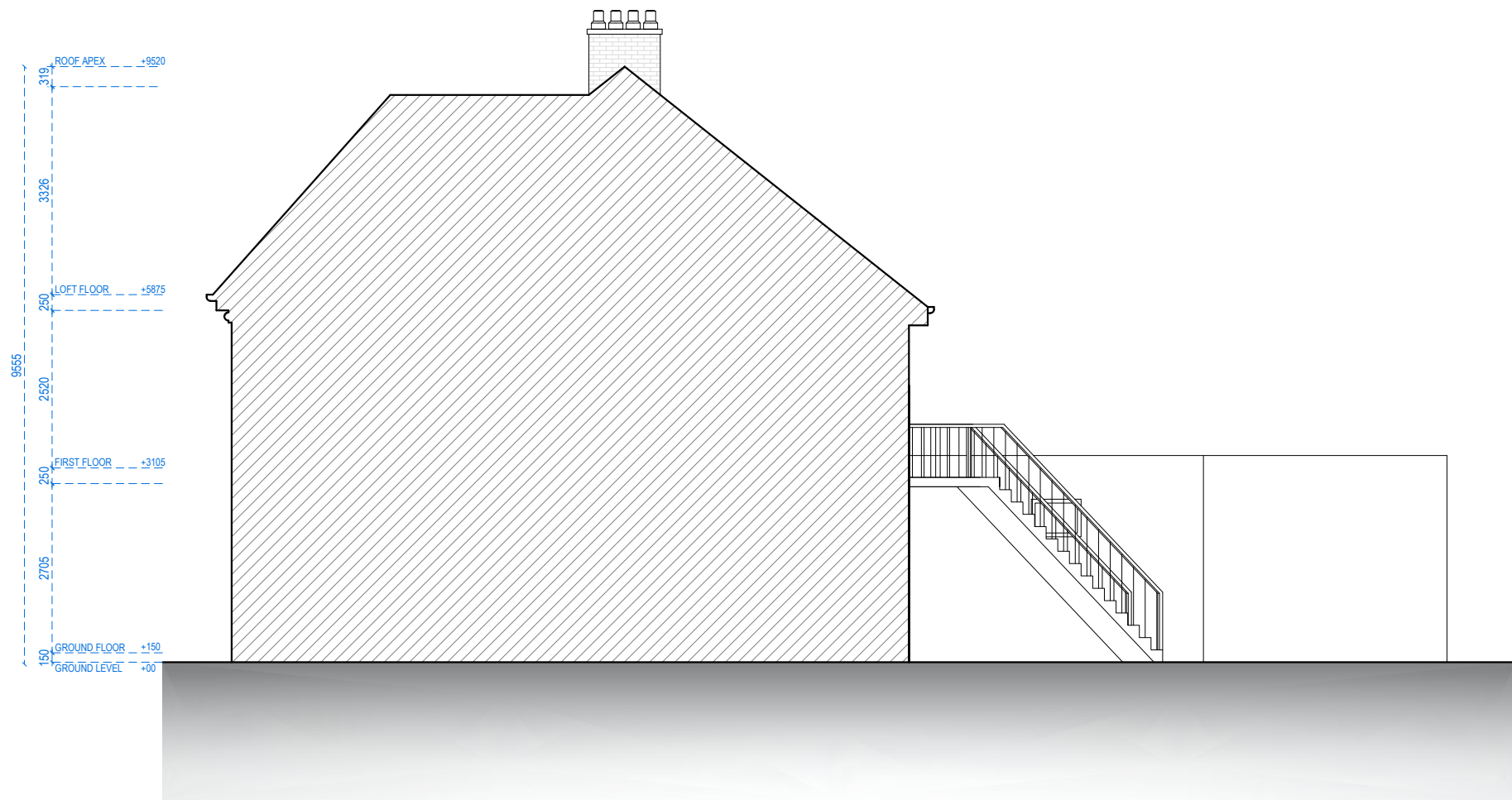
RIGHT ELEVATION
