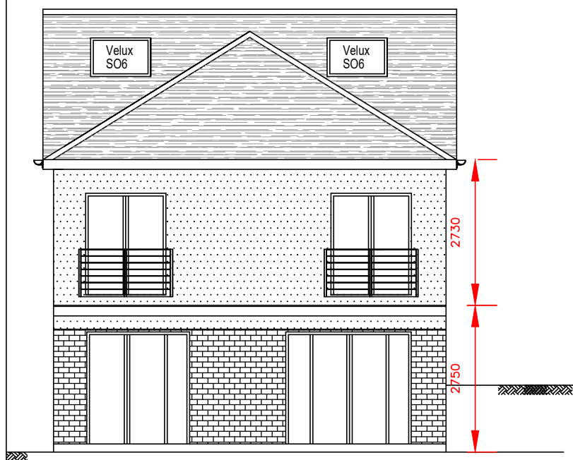
OPTION-4 REAR ELEVATION Scale:-1:100
