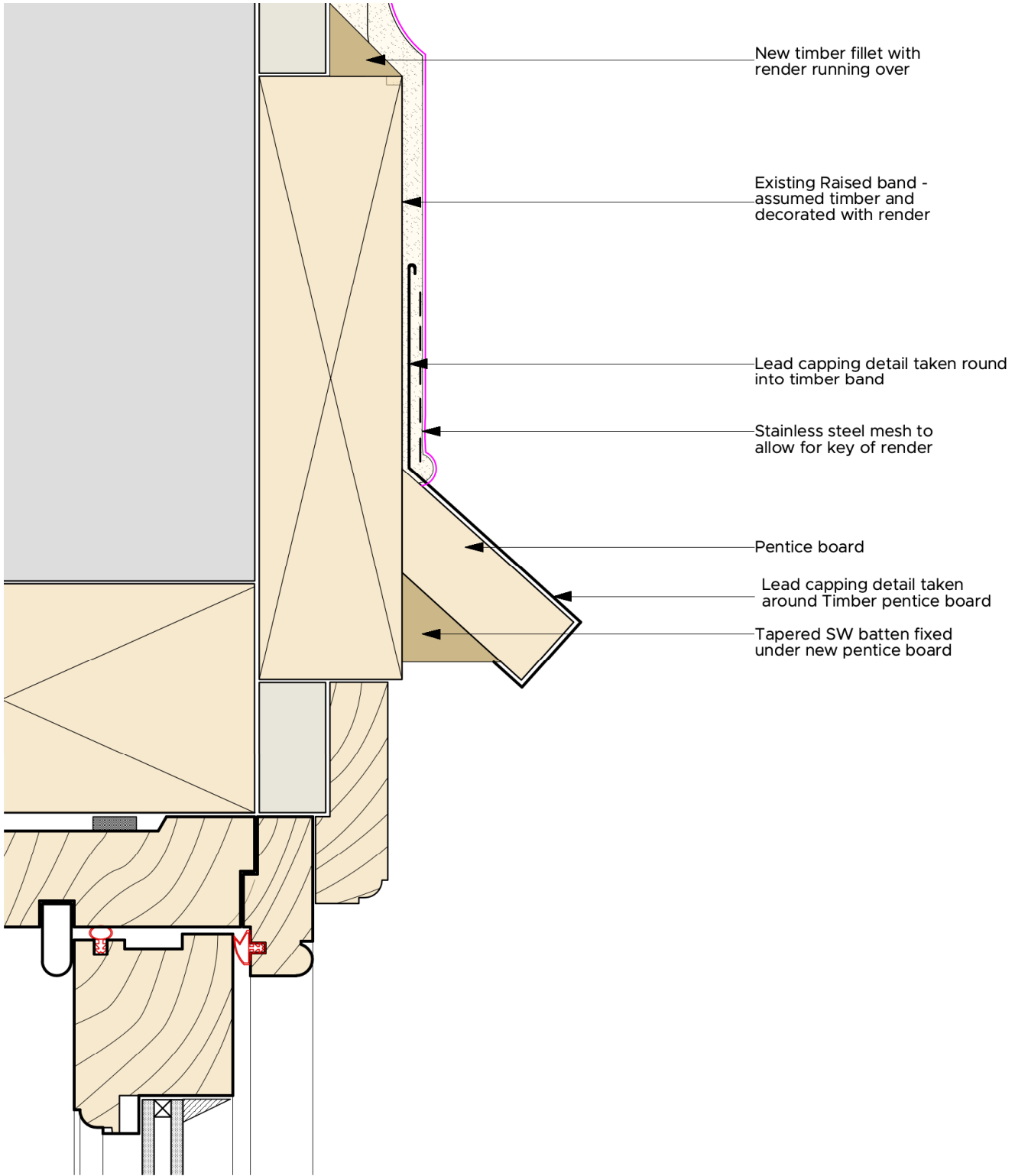
DETAIL A-A
