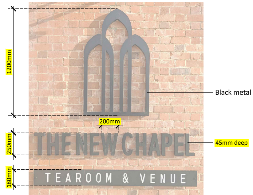
Signage dimensions
