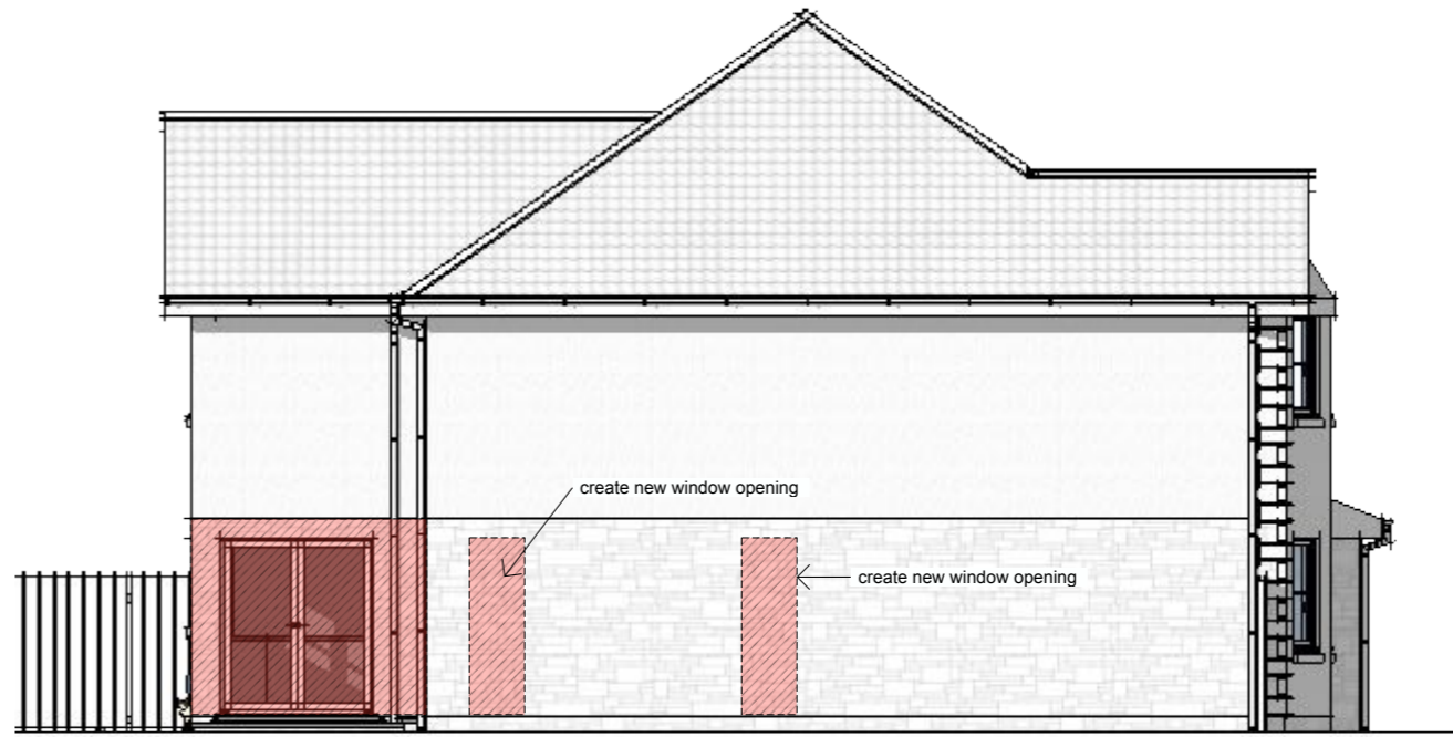
E :: EXISTING SIDE ELEVATION 2 scale: 1:100
