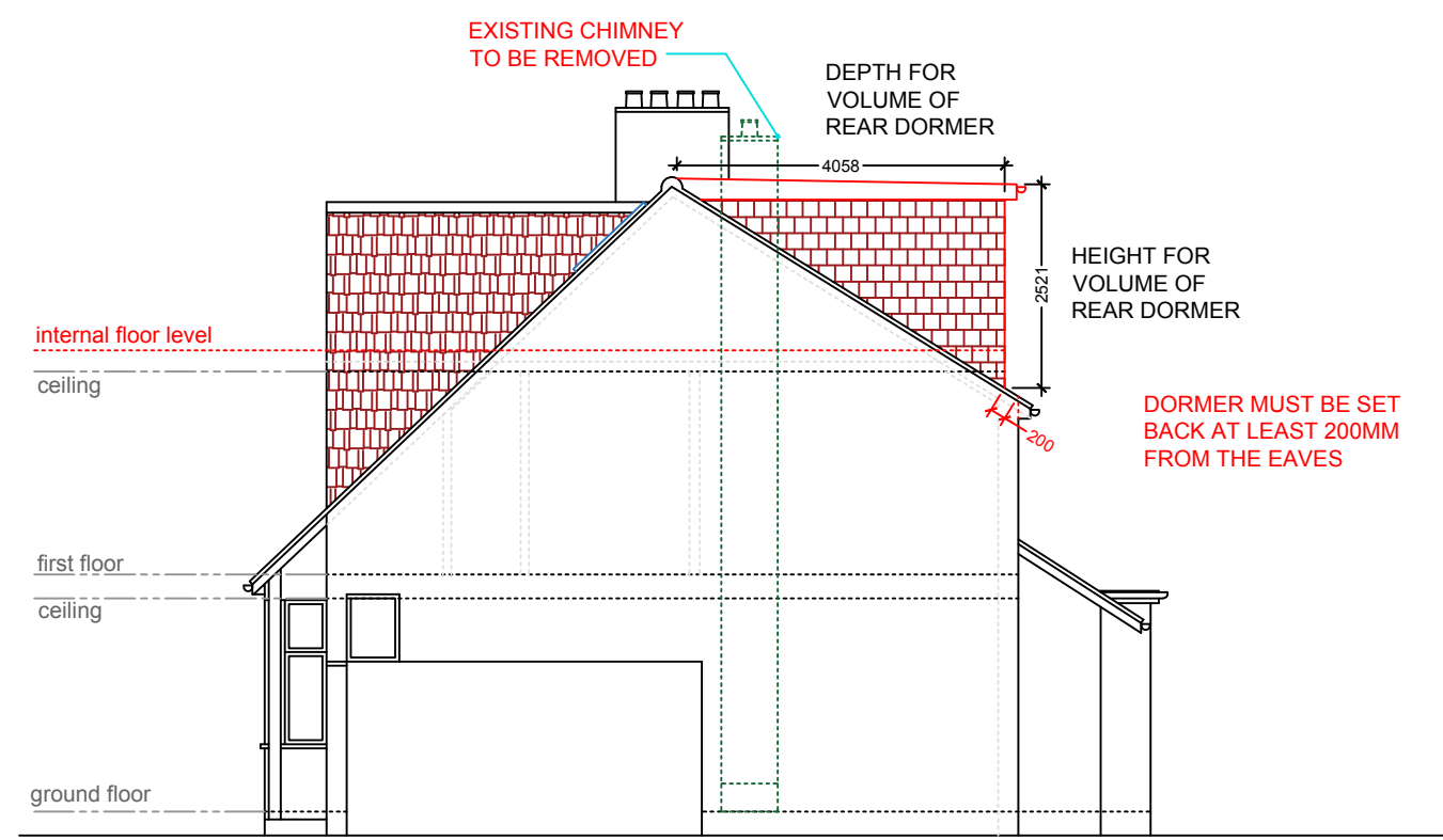
14 R.H.SIDE ELEVATION - EXISTING 1:100
