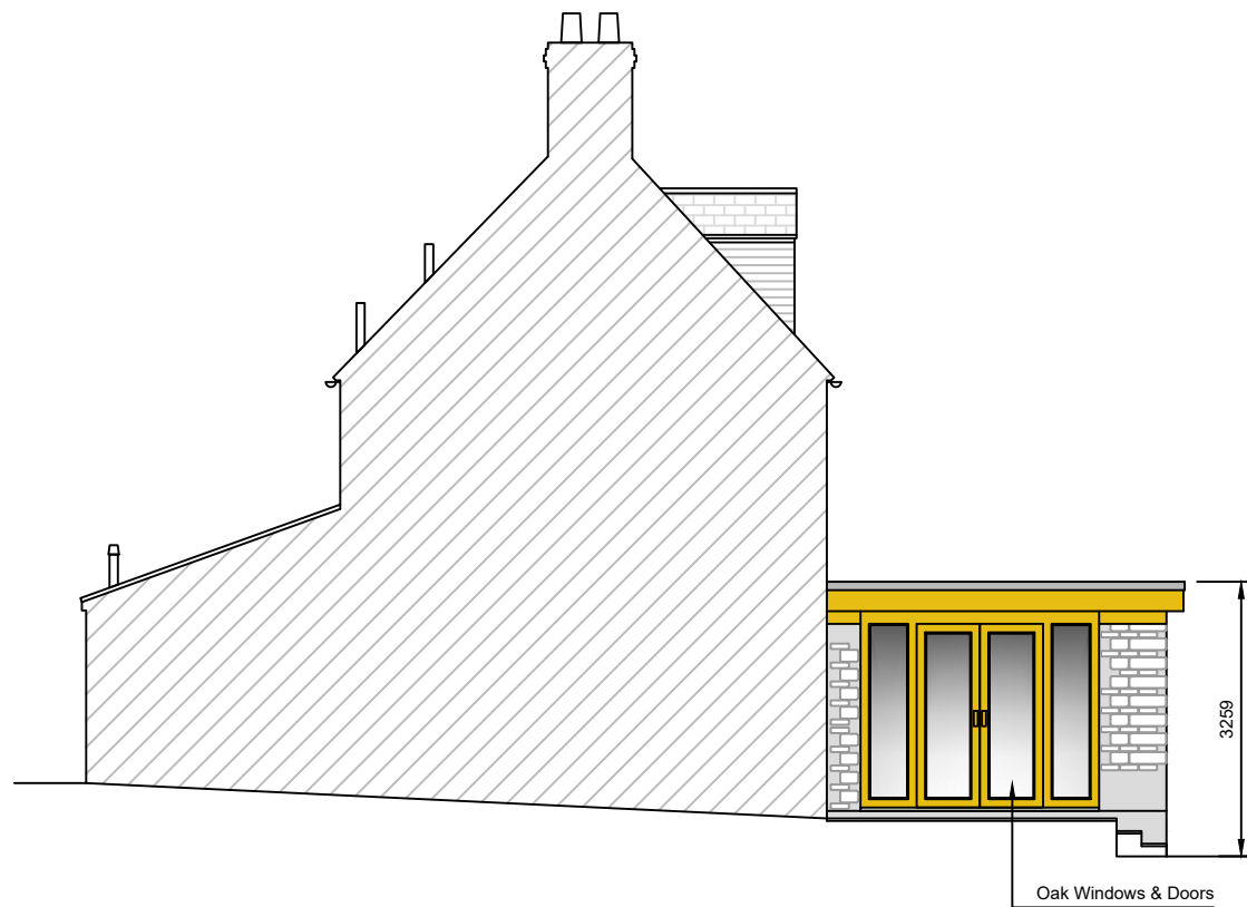
RIGHT ELEVATION
