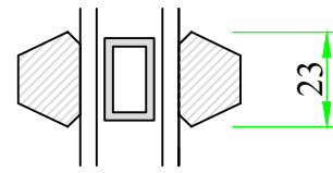
Glazing Bar
