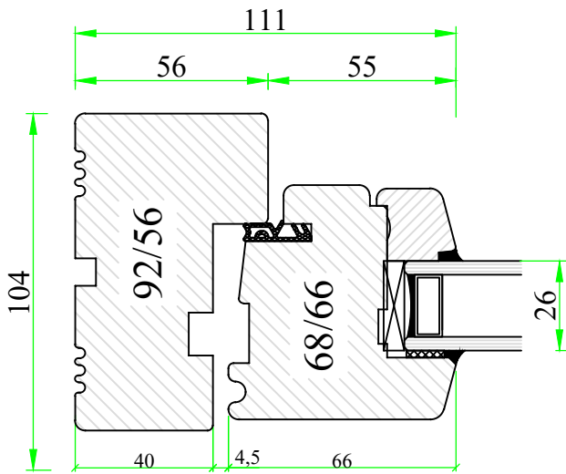
Frame Side / Jamb
