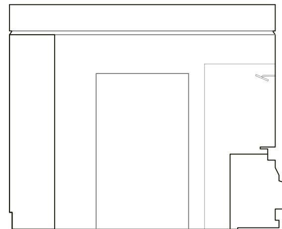
ELEVATION 04 - ENSUITE
