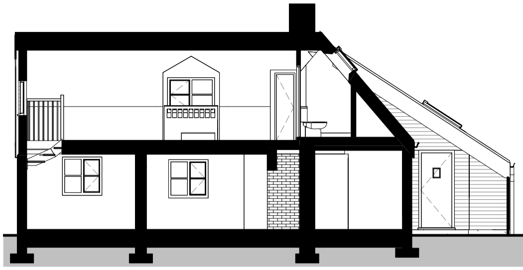
A Existing Section A 1 : 100
