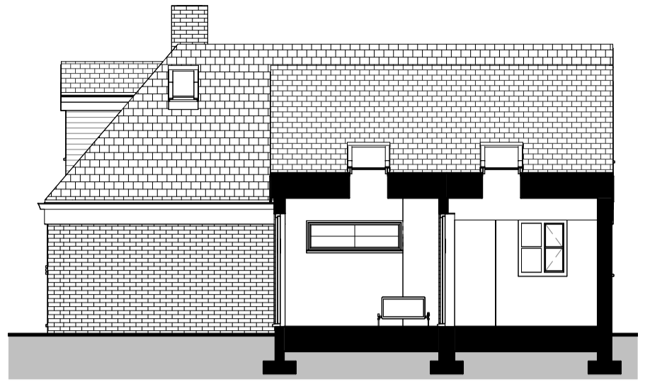
B Existing Section B 1 : 100
