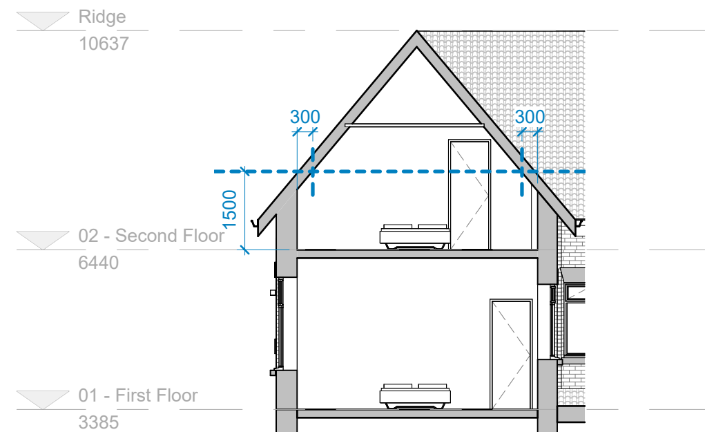
Section 02 1 : 100
