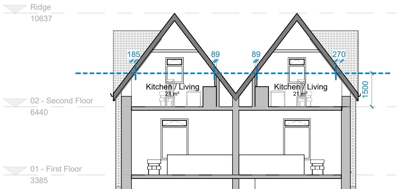
Section 01 1 : 100
