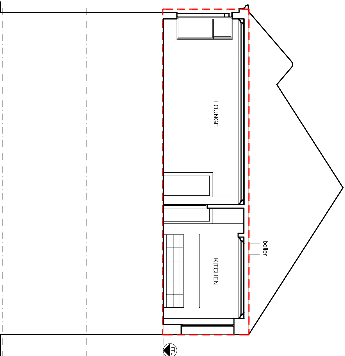
SECTION A-A 1:100
