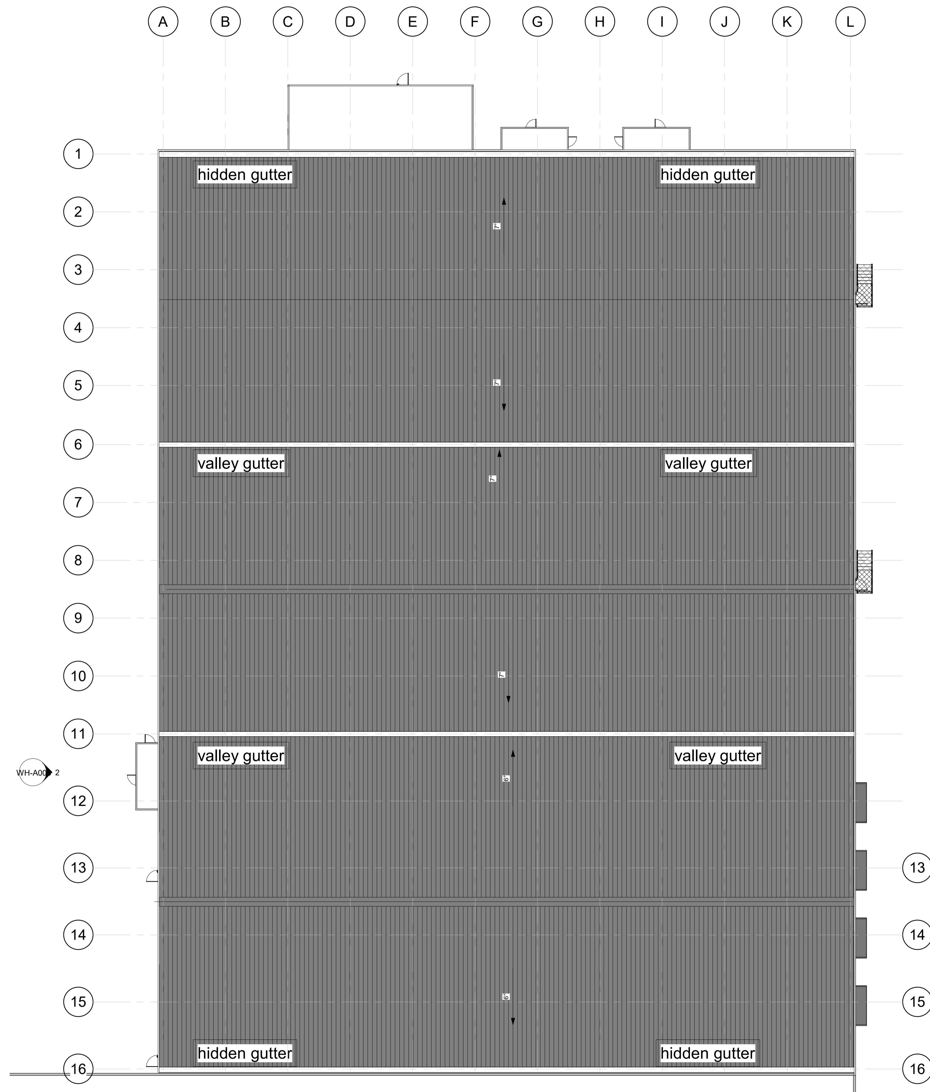
1 Roof 1 : 200
