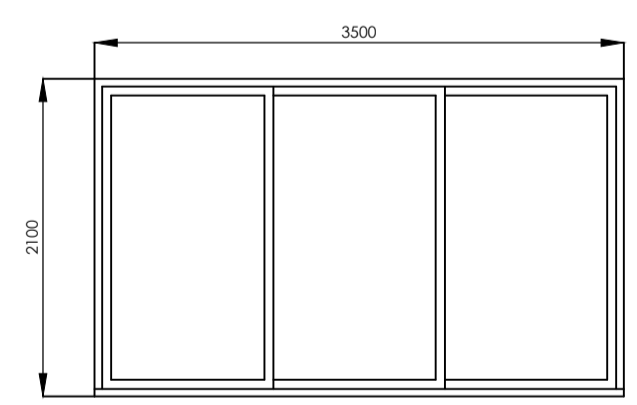
DOOR DETAILS
