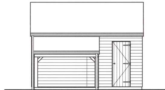
Right Elevation
