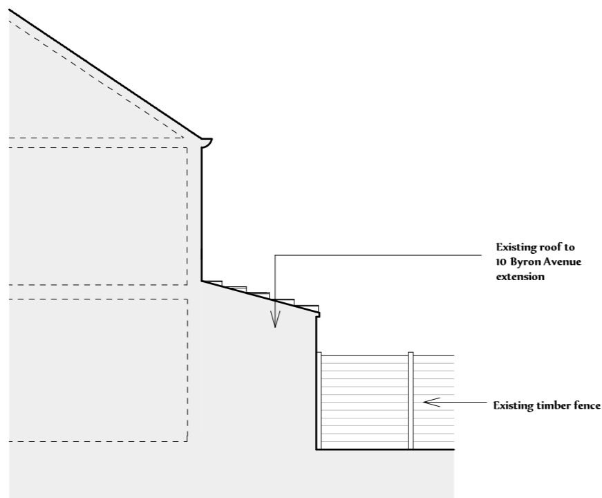
EXISTING ELEVATION FROM 10 BYRON AV SCALE 1:100 @ A3
