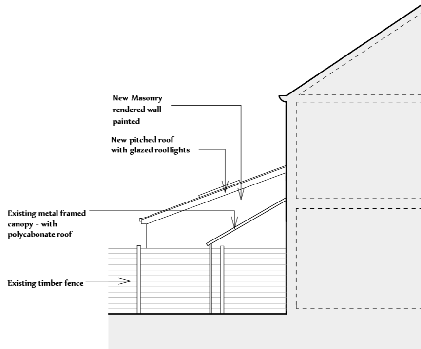
PROPOSED ELEVATION FROM 14 BYRON AV SCALE 1:100 @ A3
