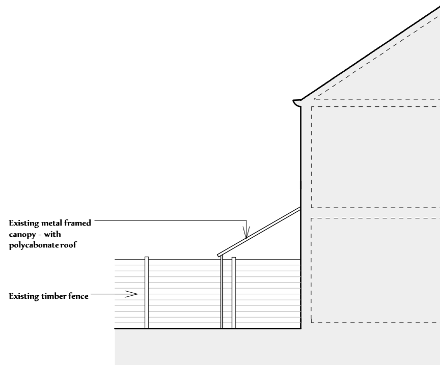
EXISTING ELEVATION FROM 14 BYRON AV SCALE 1:100 @ A3
