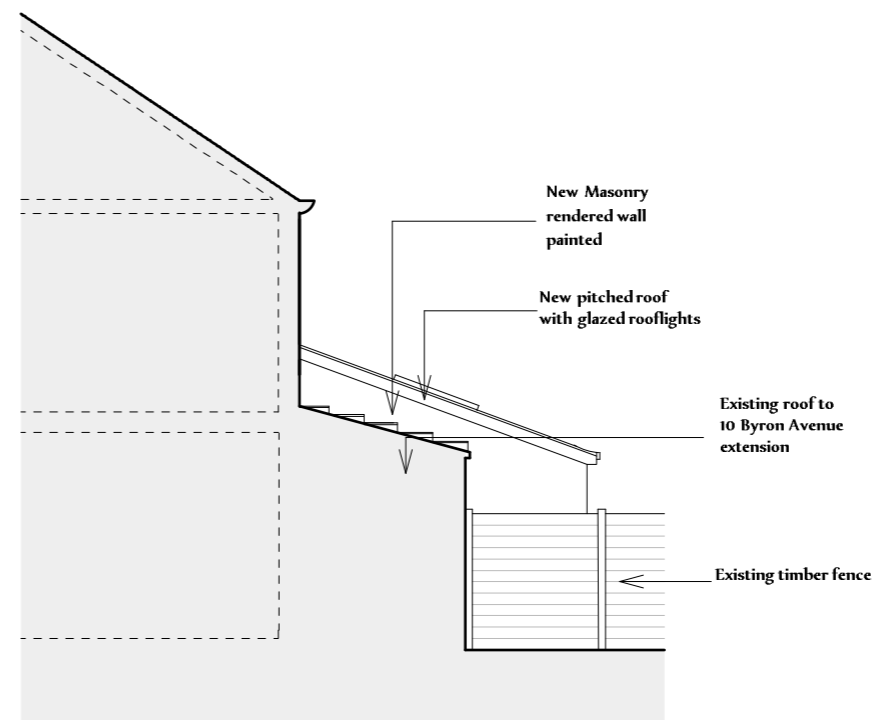
PROPOSED ELEVATION FROM 10 BYRON AV SCALE 1:100 @ A3
