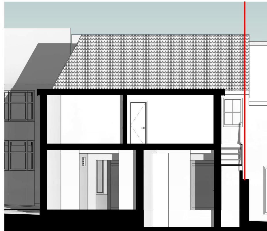
2 | EXISTING A-A SECTION 1 : 100
