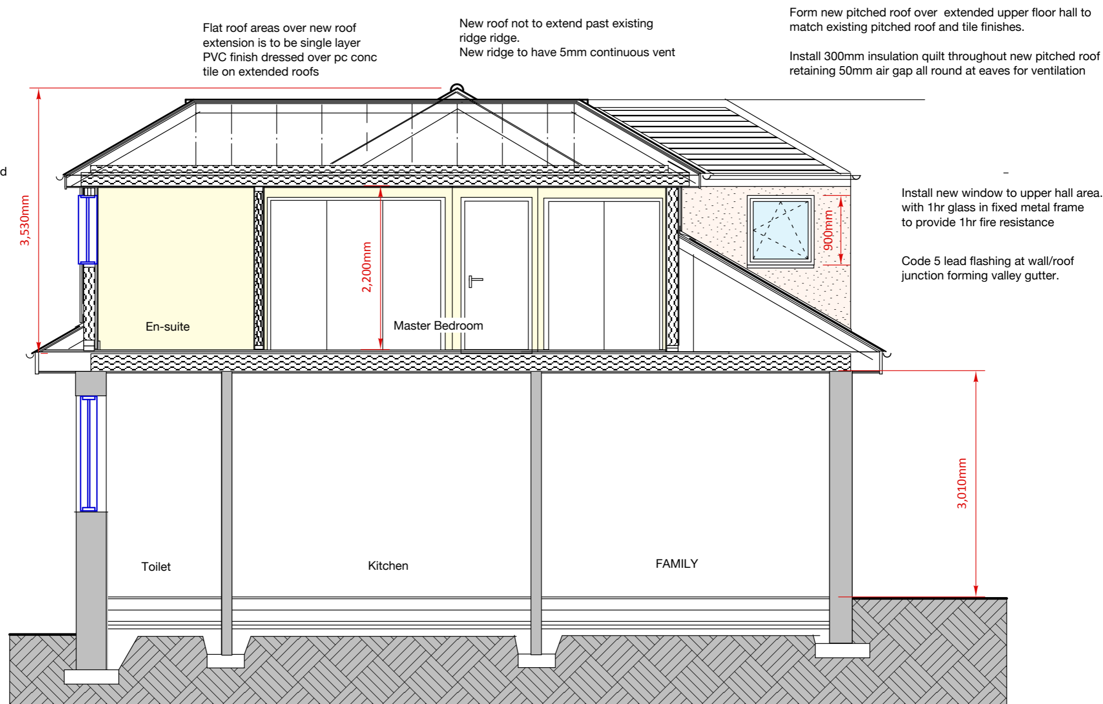
SECTION A-A...
