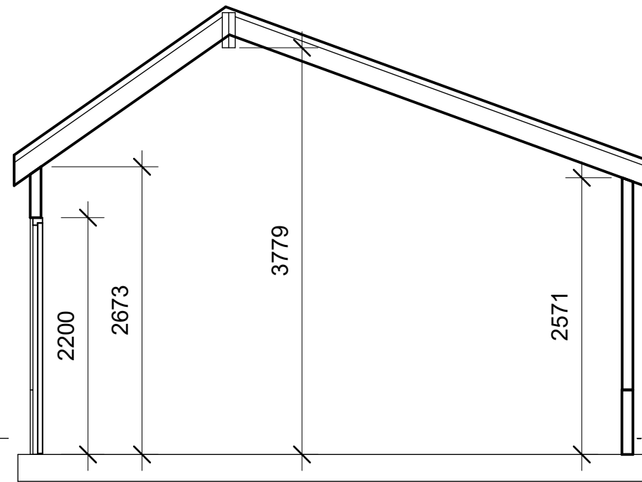
1 Section 1 1 : 50
