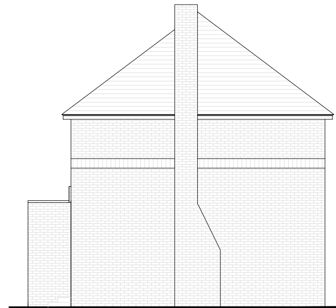
NE ELEVATION
