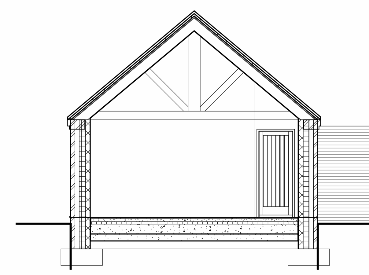
5 SECTION UNITS 8 1 : 50
