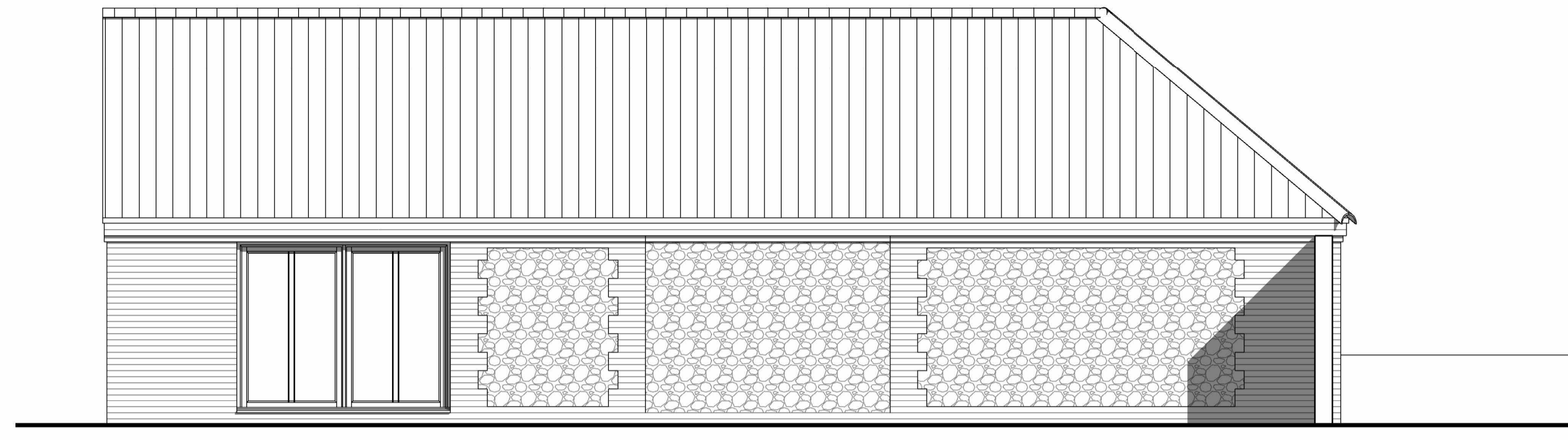
2 WEST ELE UNIT 8 PRO 1 : 50
