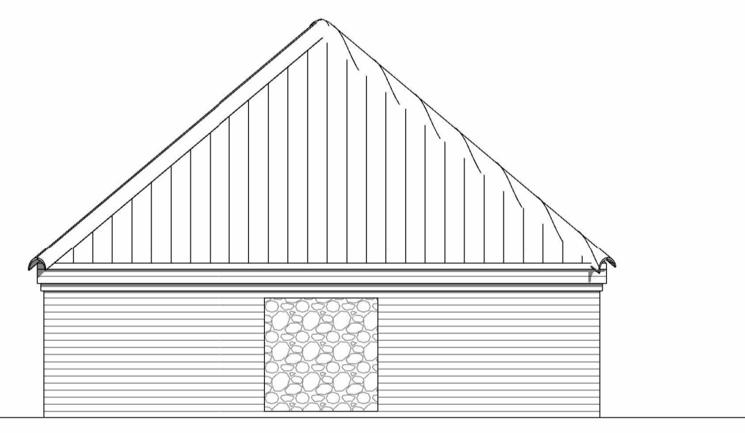
4 SOUTH ELE UNIT 8 PRO 1 : 50
