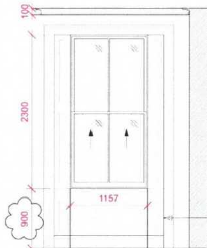
W03 GUEST BEDROOM WINDOW Scale: 1:40
