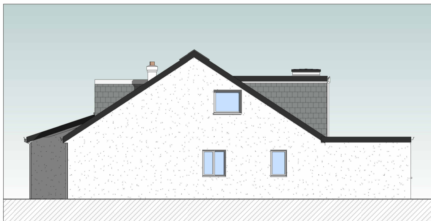
D ELEVATION D 1:100
