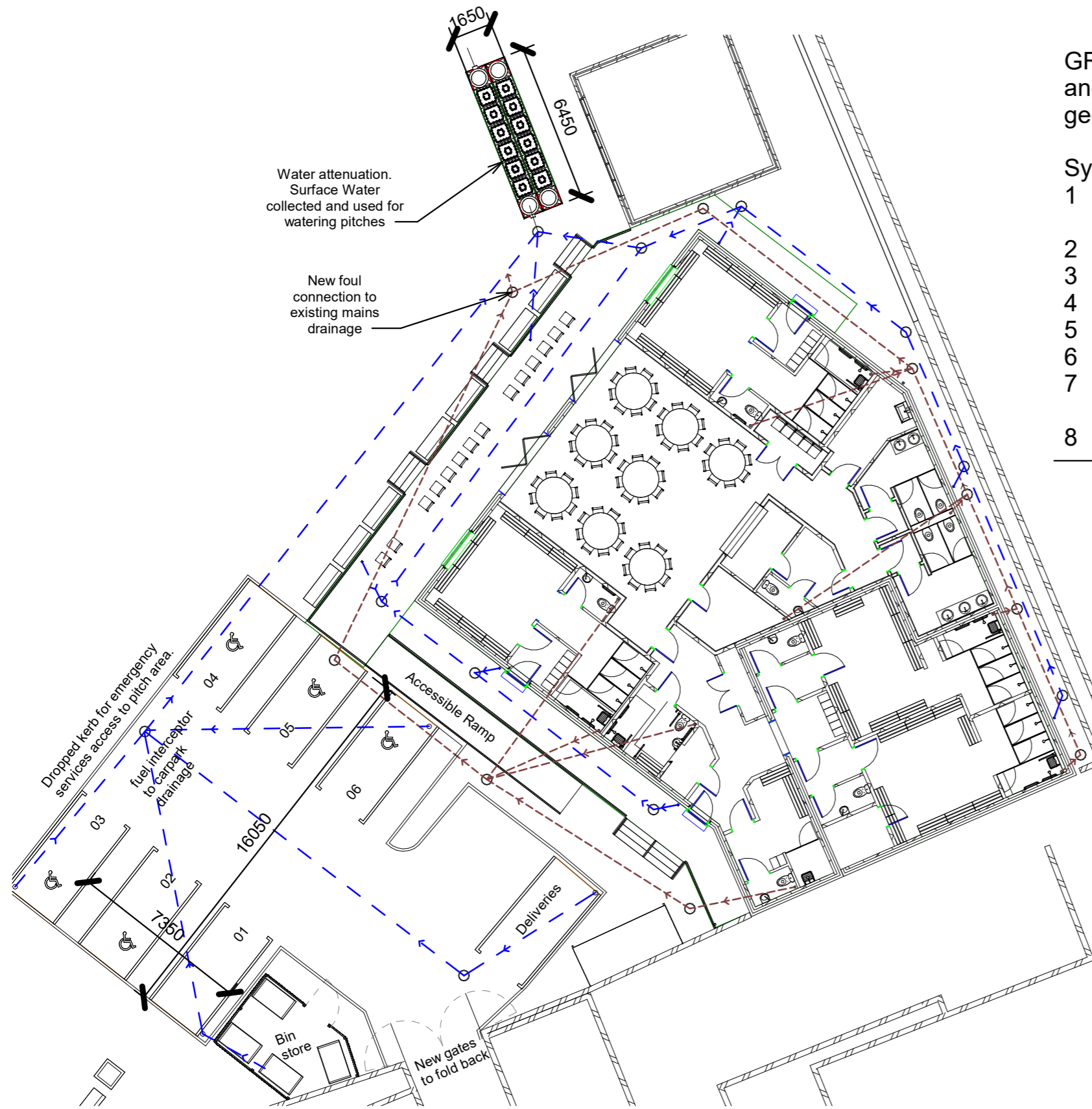
1 Drainage Layout 1 : 200
