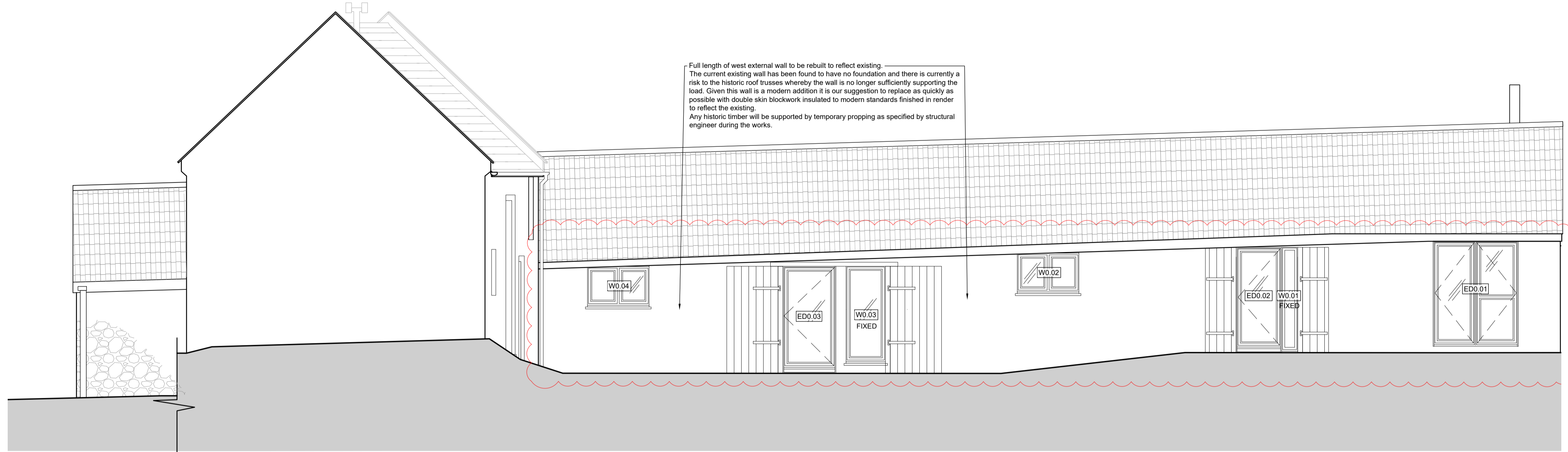
ELEVATION 1
