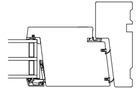
Jamb Detail 1:5
