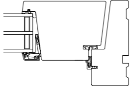
Jamb Detail 1:5
