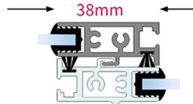
Box interlock
