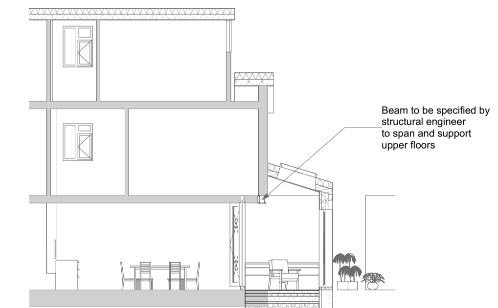
Section 01 @1:100
