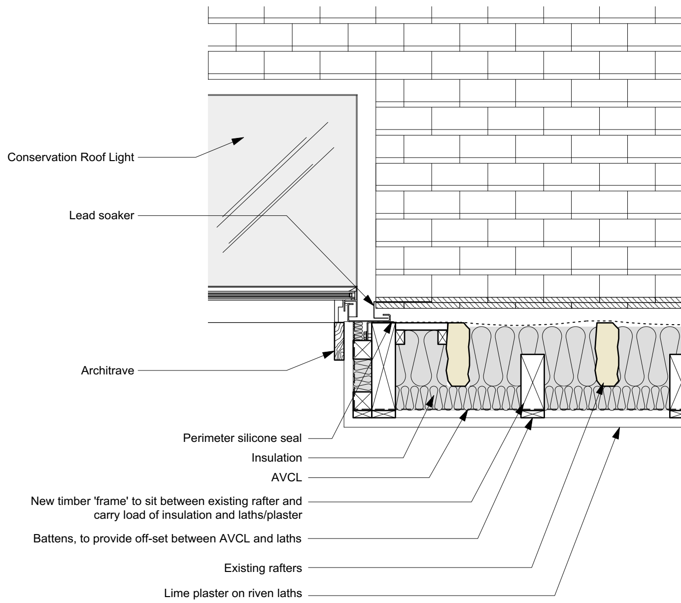
02 603 DETAIL A-A SECTION 1:10
