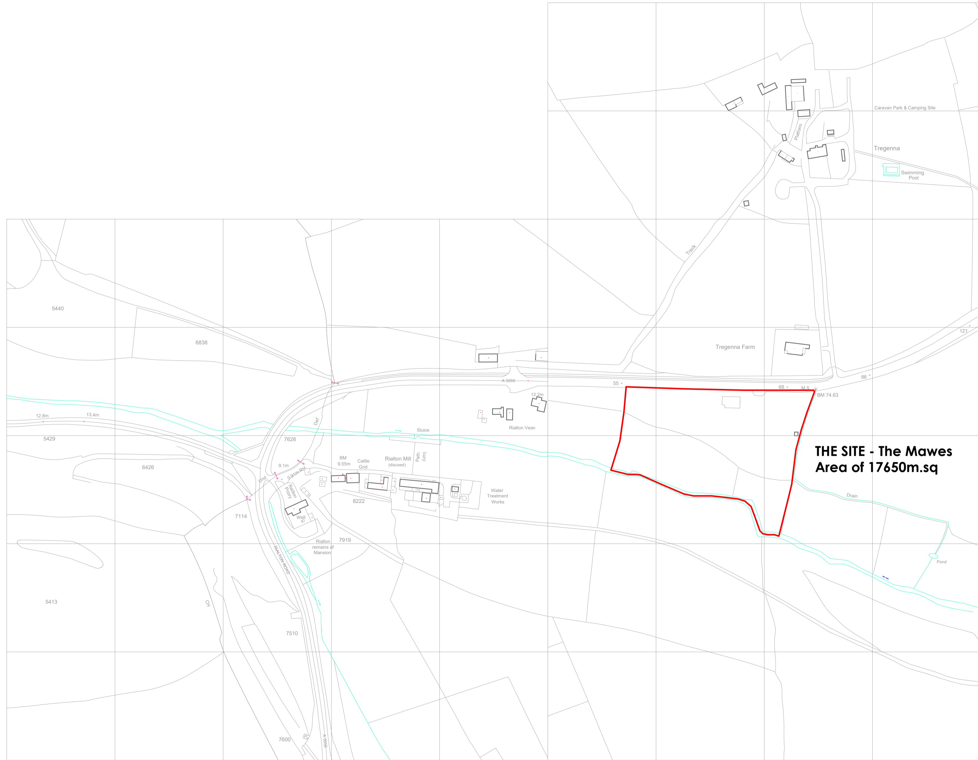
1 OS Plan 1 : 2000
