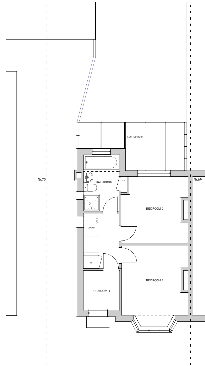
2 1F Plan Scale: 1:100
