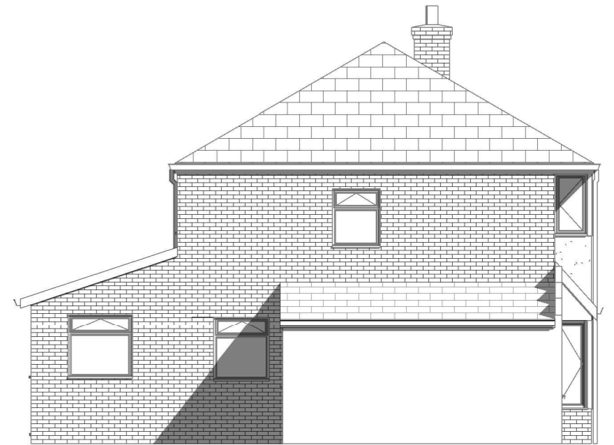
4 Gable 1 : 100
