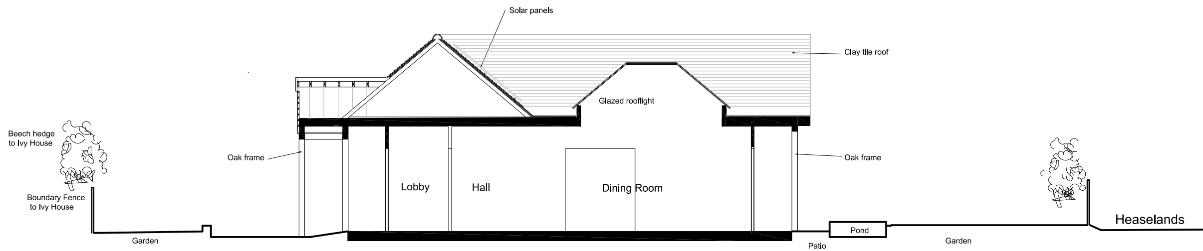
Section E - E
