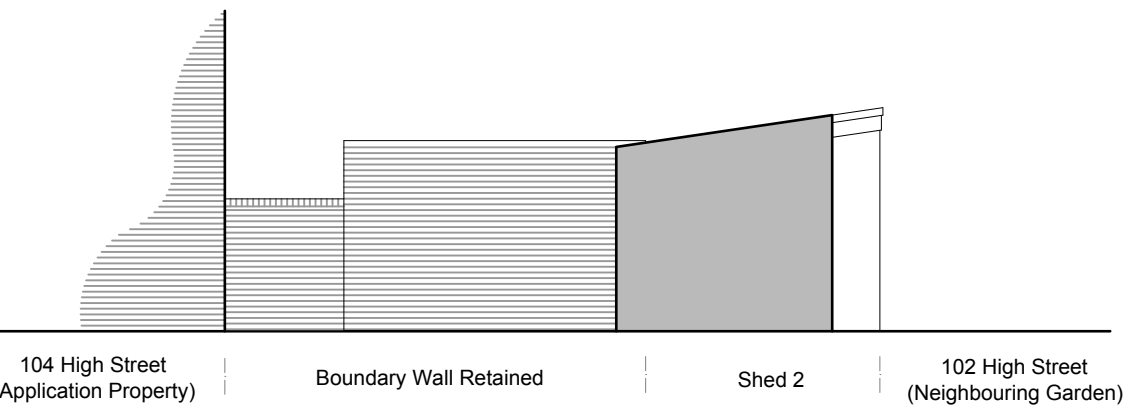
ELEVATION 3
