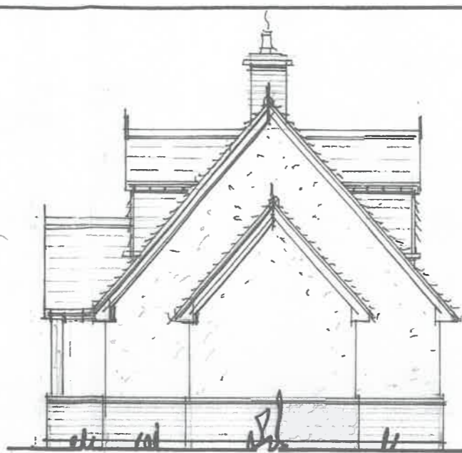
end elevation 1:100
