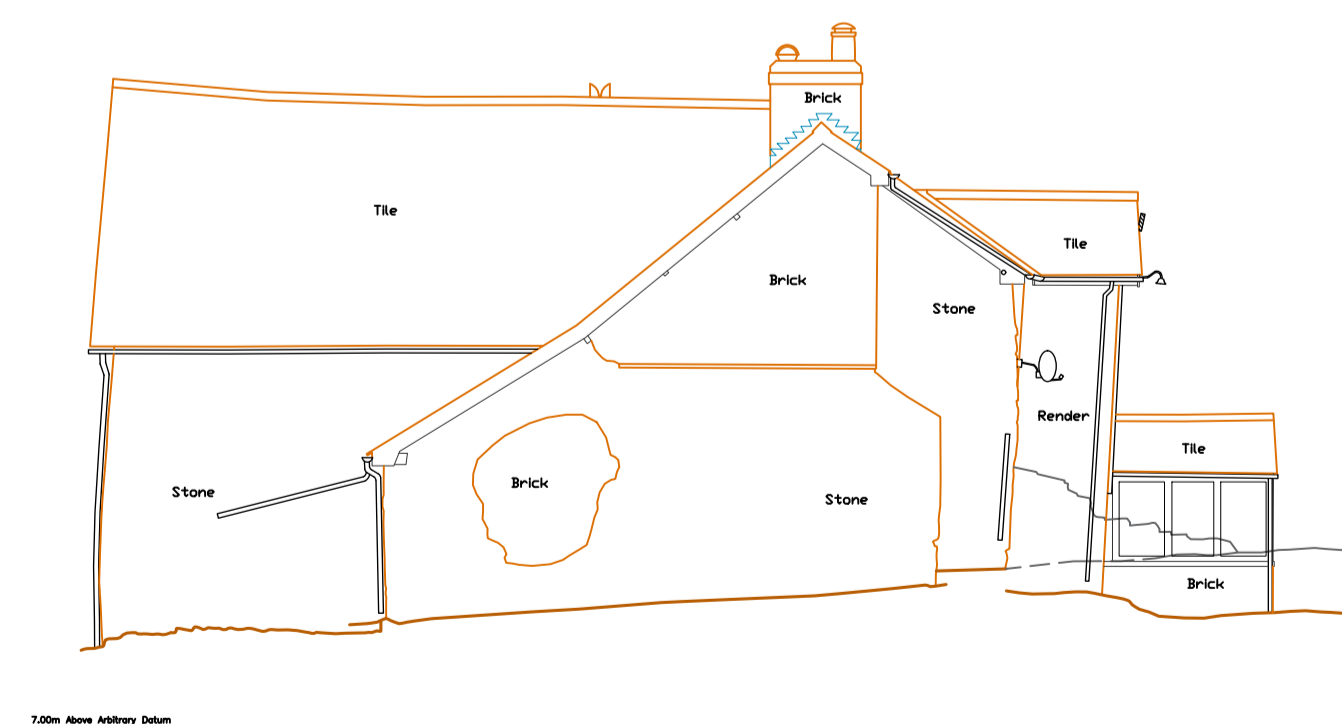
ELEVATION 4
