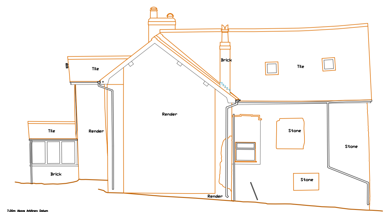
ELEVATION 2
