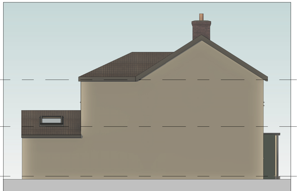
4 East 1 : 100
