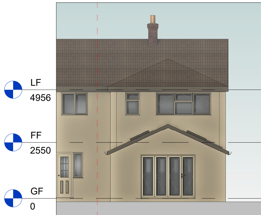
3 South 1 : 100
