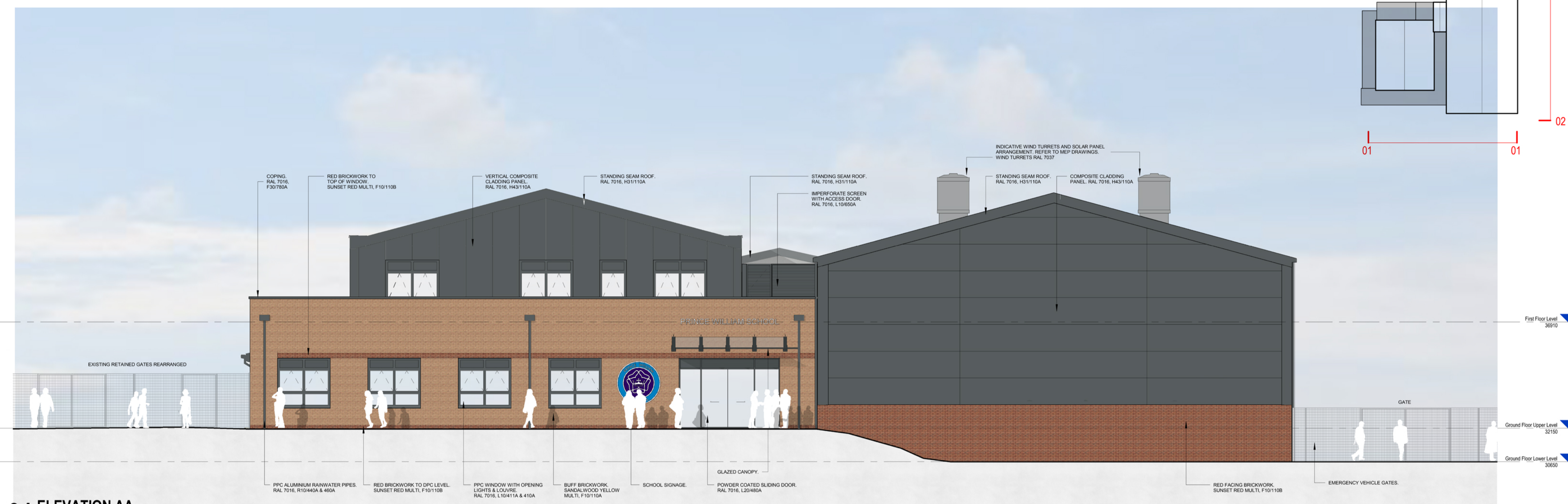
01 ELEVATION AA 1:100
