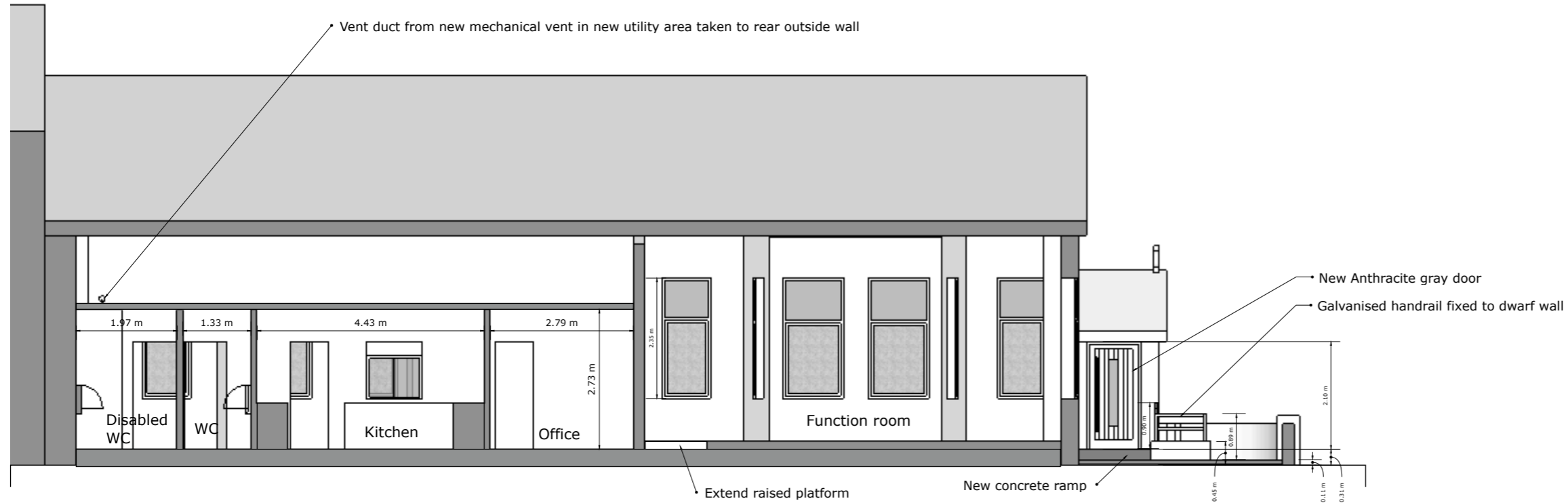
Section A-A
