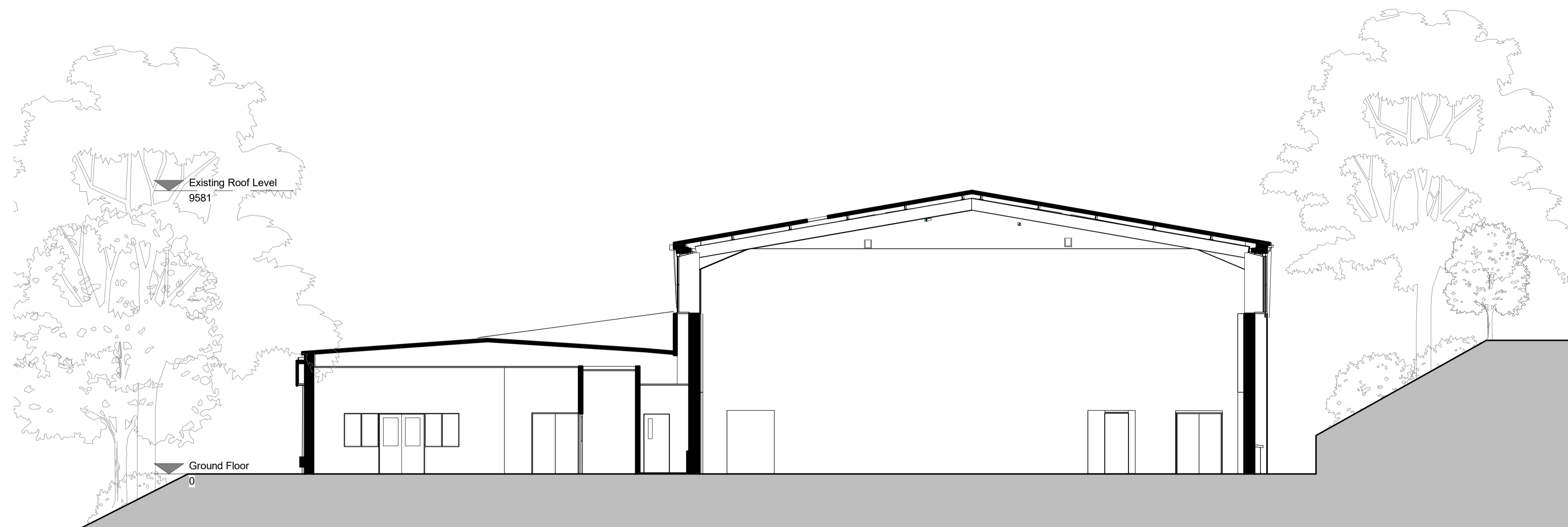
1 Existing Section AA 1 : 100
