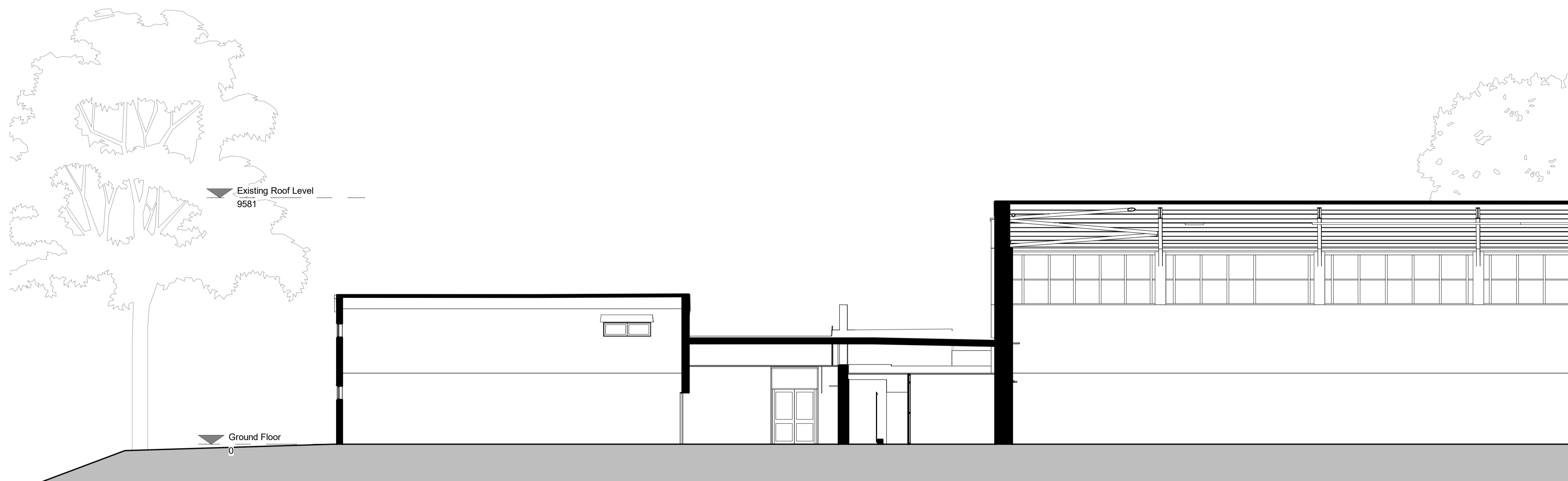
2 Existing Section BB 1 : 100
