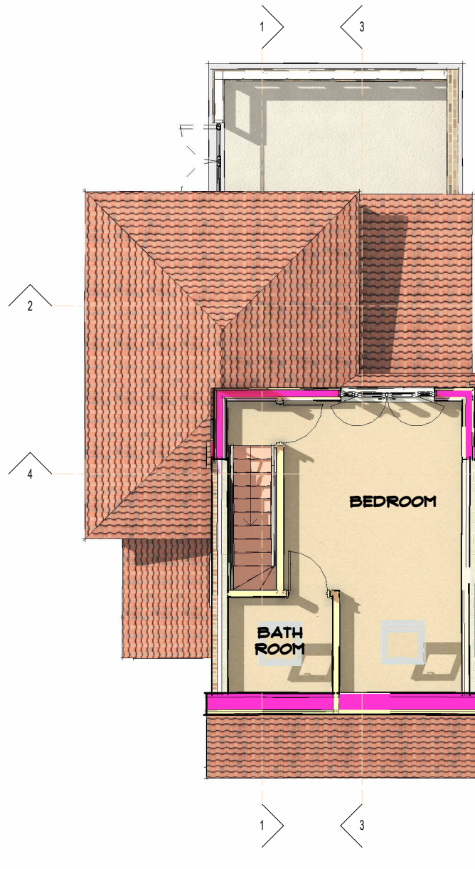
LF PRO. LOFT FLR. SCALE 1 : 100
