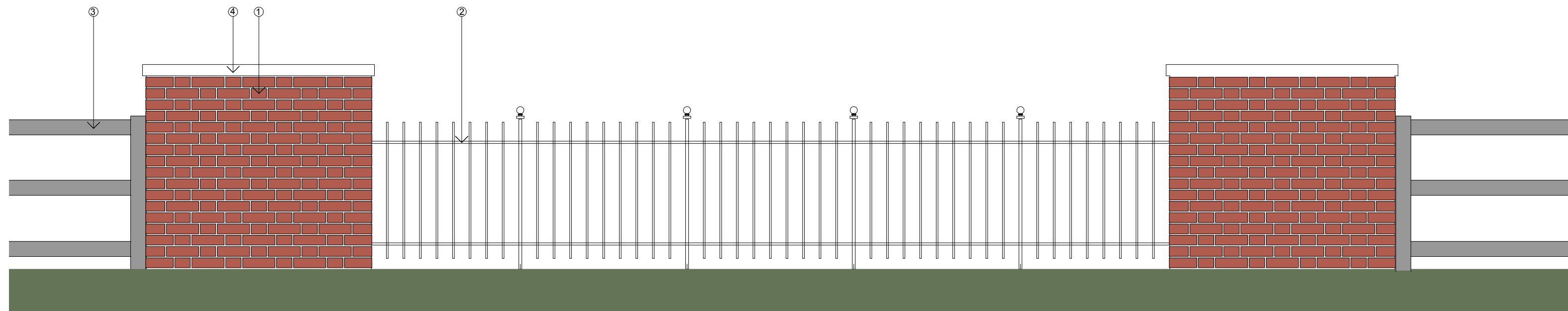
ELEVATION
